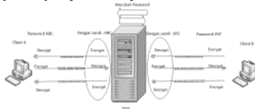
Gambar 16. Skema Komunikasi Data Enkripsi User ke User
