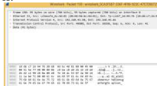
Gambar 19. Capture Pengiriman Data Login
