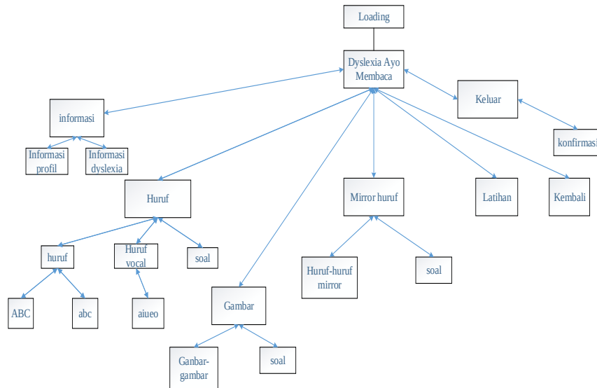
Gambar 6. Struktur Navigasi
