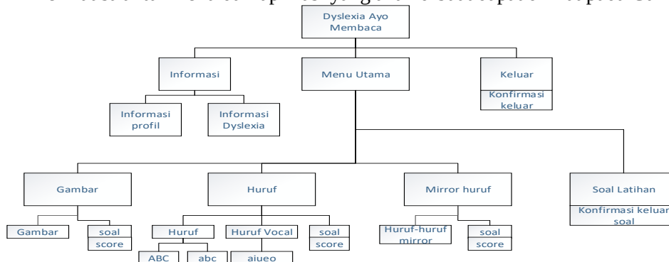
Gambar 5. Struktur Menu
