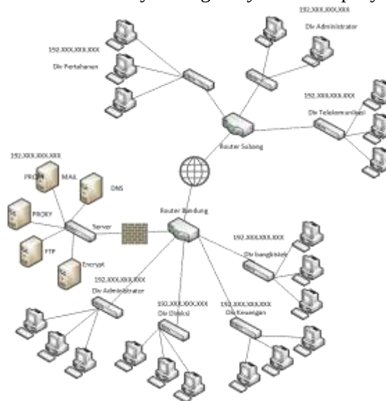
Gambar 1. Skema Jaringan
