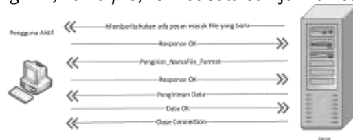
Gambar 14. Skema Komunikasi Penerimaan File
