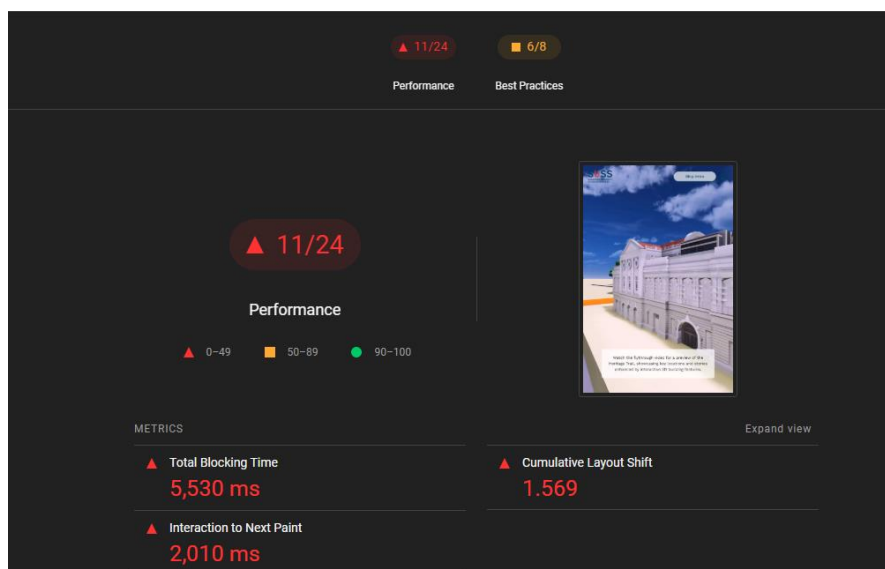
Gambar 6. Hasil Pengujian Lighthouse pada Chrome
