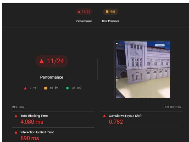
Gambar 7. Hasil Pengujian Lighthouse pada Edge
