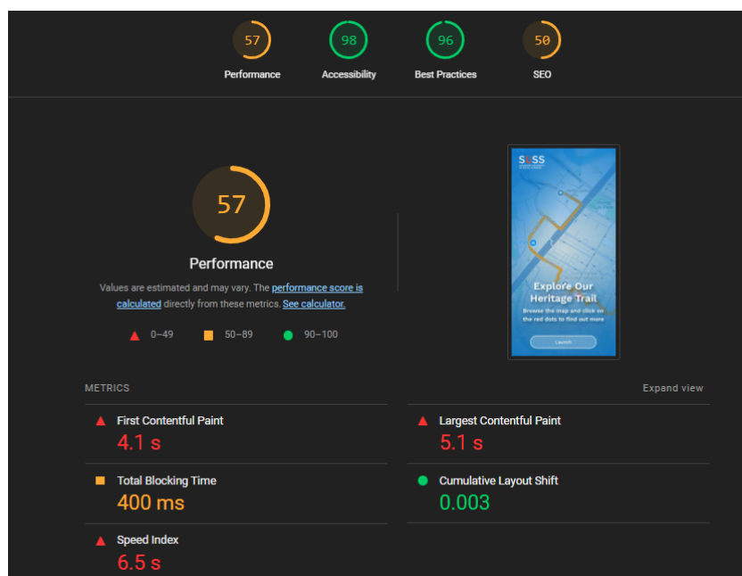
Gambar 8. Hasil Pengujian Lighthouse pada Firefox
