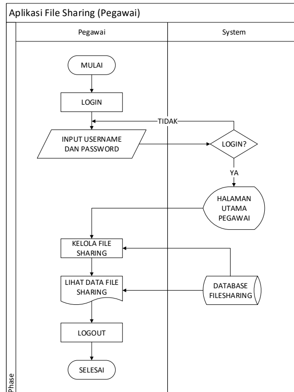
Gambar 3.3 Flowmap Sistem yang Dibangun (Pegawai)
