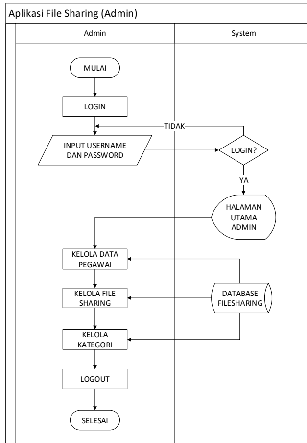
Gambar 3.2 Flowmap Sistem yang dibangun (Admin)
