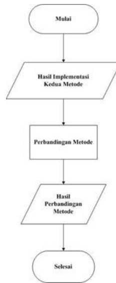
Gambar 4.1 diagram alur metode regresi linear berganda
