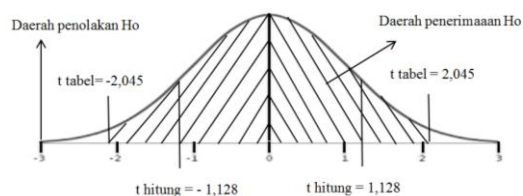
Gambar 2 Kurva Penolakan dan Penerimaan H_0
